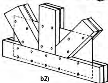
Obr. 2 Styčnická příhradového vazníku – alternativy spojení
